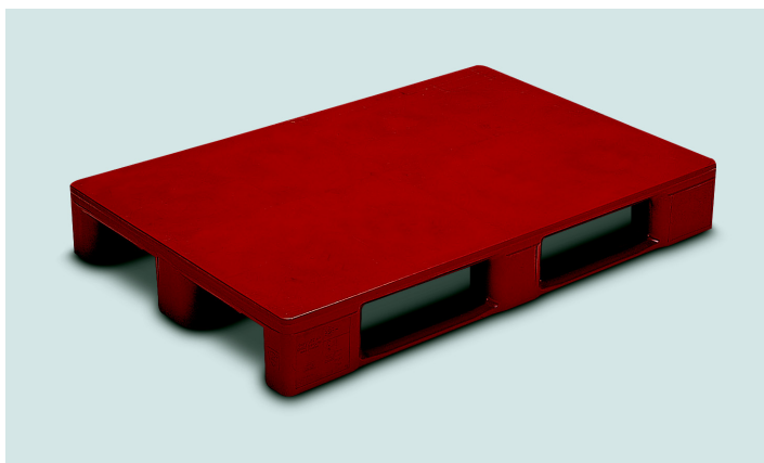
Kunststoff-Palette Euro Norm 1200 x 800 x 165 mm
